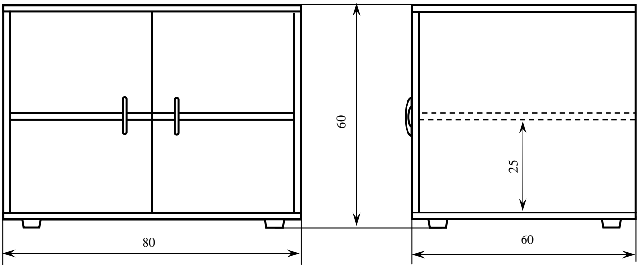
Rys.2.4. Stolik pod RTV. Oznaczenie WP8-19/09.
