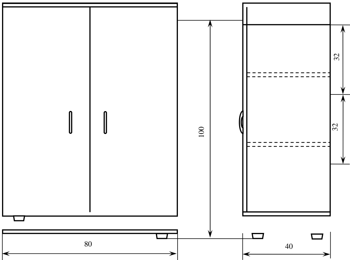
Rys.2.10. Komódka meblowa. Oznaczenie WP8-48/09.
