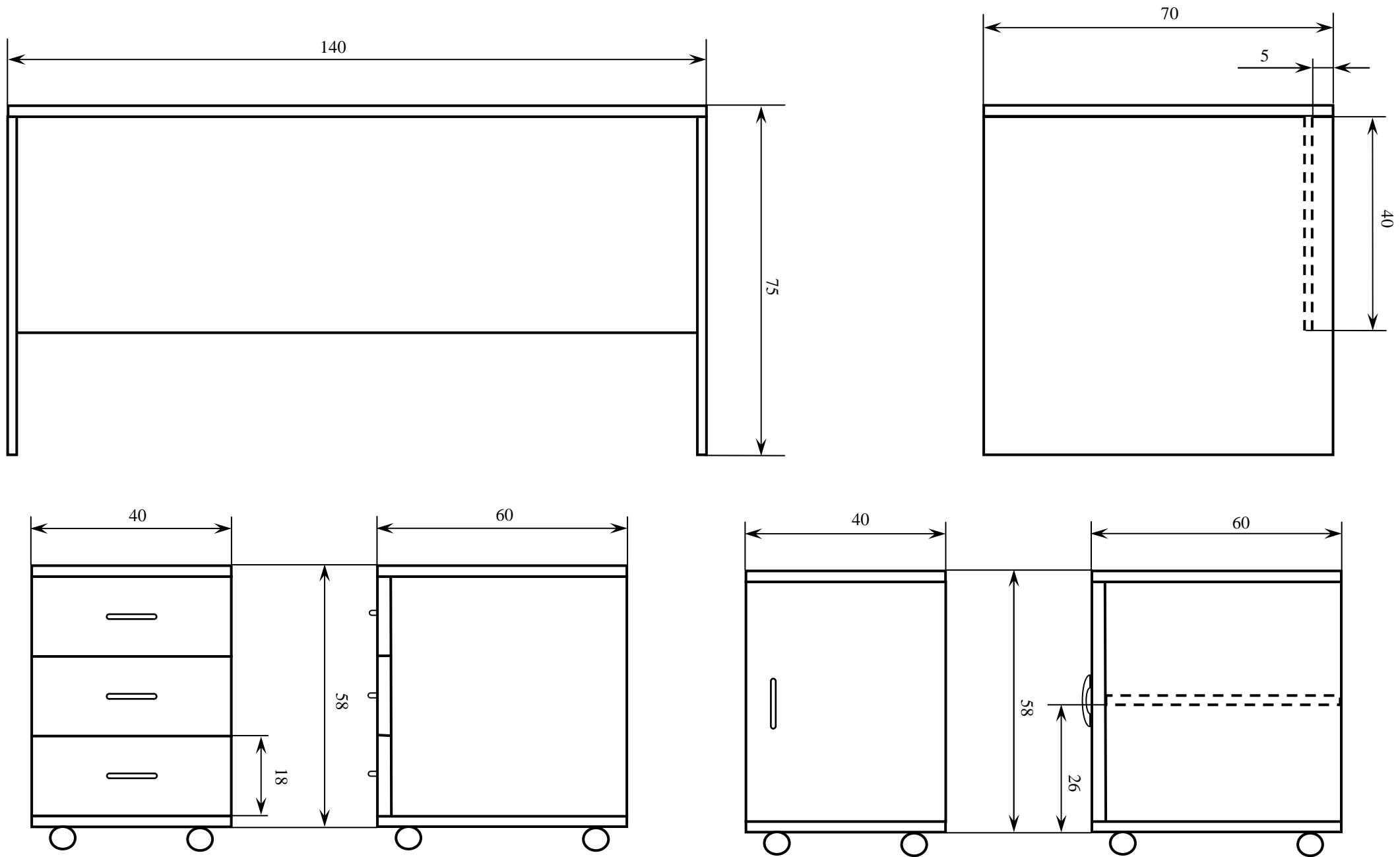
Rys.1.1. Biurko kancelaryjne z dwoma kontenerami. Oznaczenie WP1-2/09.
