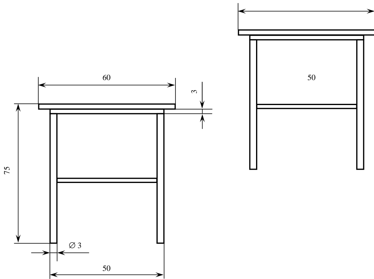
Rys.1.4. Stolik pod drukarkę na metalowej podstawie. Oznaczenie WP1-20/09.
