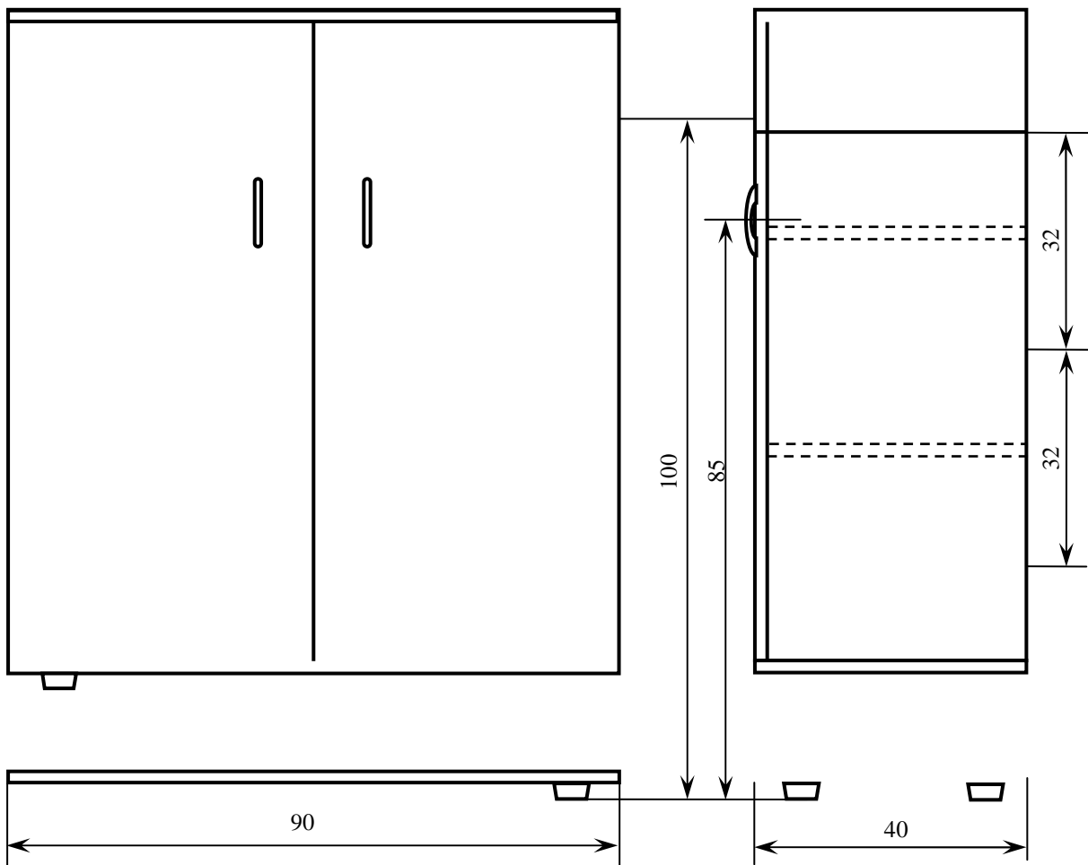
Rys.1.10. Komódka meblowa. Oznaczenie WP8-48/09.
