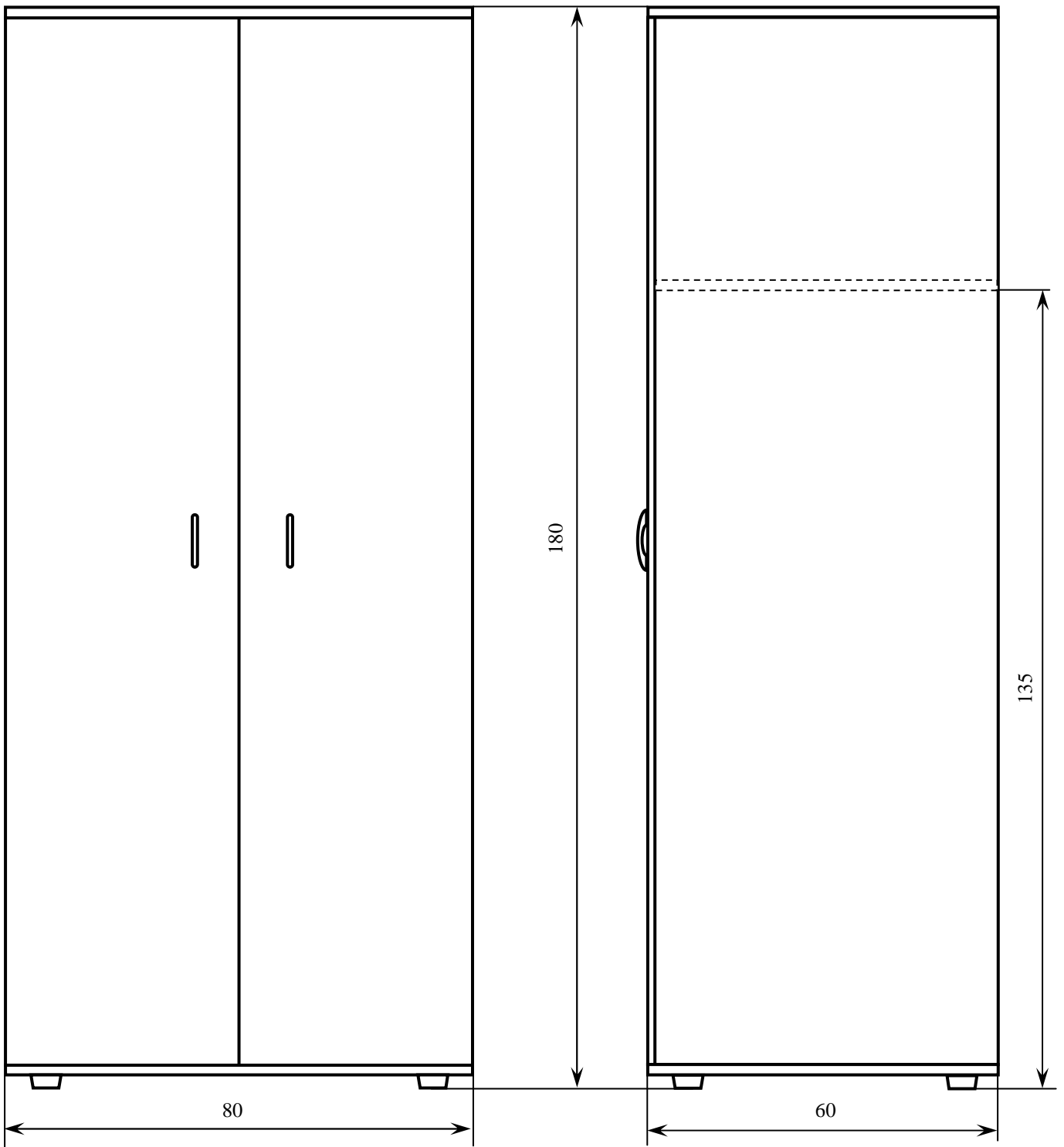
Rys.2.6. Szafa ubraniowa 2-drzwiowa gabinetowa. Oznaczenie WP8-27/09.
