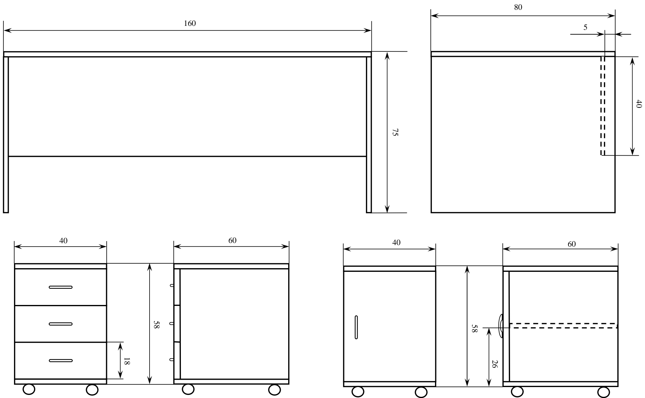
Rys.2.3. Biurko gabinetowe z dwoma kontenerami. Oznaczenie WP8-2/09.
